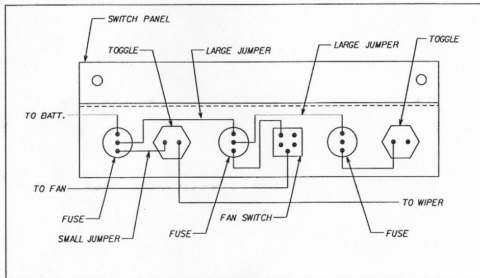
OPTIONAL CAB WIRING
